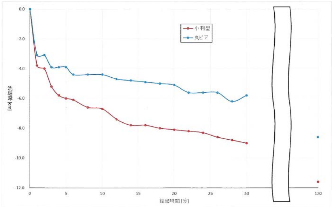
図-2 洗掘深経時変化図
