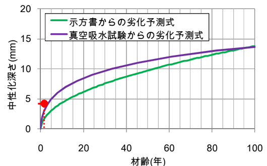
図-6 示方書と真空吸水試験による劣化予測式の関係
