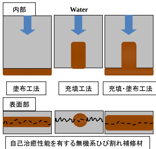
図-1 補修工法のイメージ
