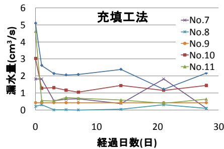
図-3 通水試験結果(充填工法)
