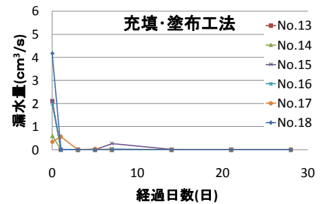
図-4 通水試験結果(充填・塗布工法)
