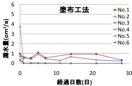
図-2 通水試験結果(塗布工法)
