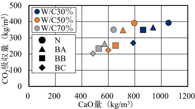
図-1 CaO 量と CO 2 吸収量の関係
