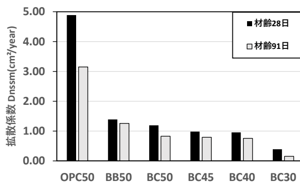
図-2 24 時間における拡散係数
