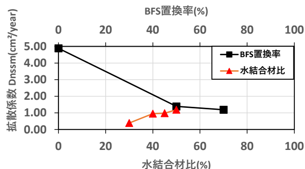
図-3 BFS 配合の材齢 28 日における 2 つの要因 (上軸:水結合材比,下軸:BFS 置換率)と拡散係数の関係
