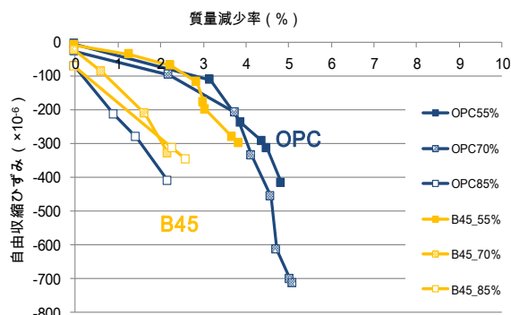
図-3 自由収縮ひずみと質量減少率
