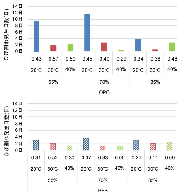
図-5 拘束度とひび割れ日数
