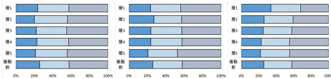
図-4 配合②に置ける振動締め後の材料構成割合 (左から順に 3 秒, 10 秒, 60 秒)
