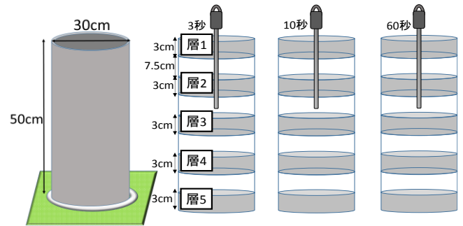
図-1 鉛直締固め試験概要図
