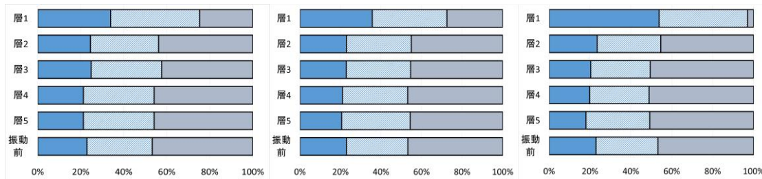
図-3 配合①に置ける振動締め後の材料構成割合 (左から順に 3 秒, 10 秒, 60 秒)
