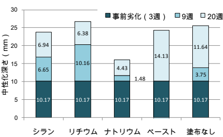
図-4 既設・中性化促進試験
