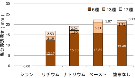
図-3 新設・塩水浸漬試験
