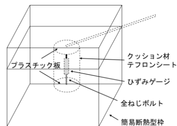
図-1 コンクリート簡易断熱装置概要
