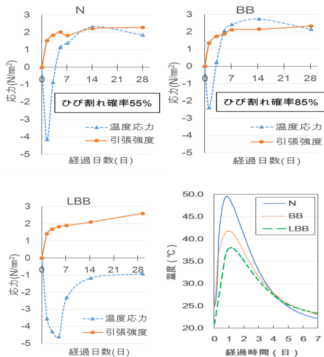
図-2 引張強度と温度応力による比較
