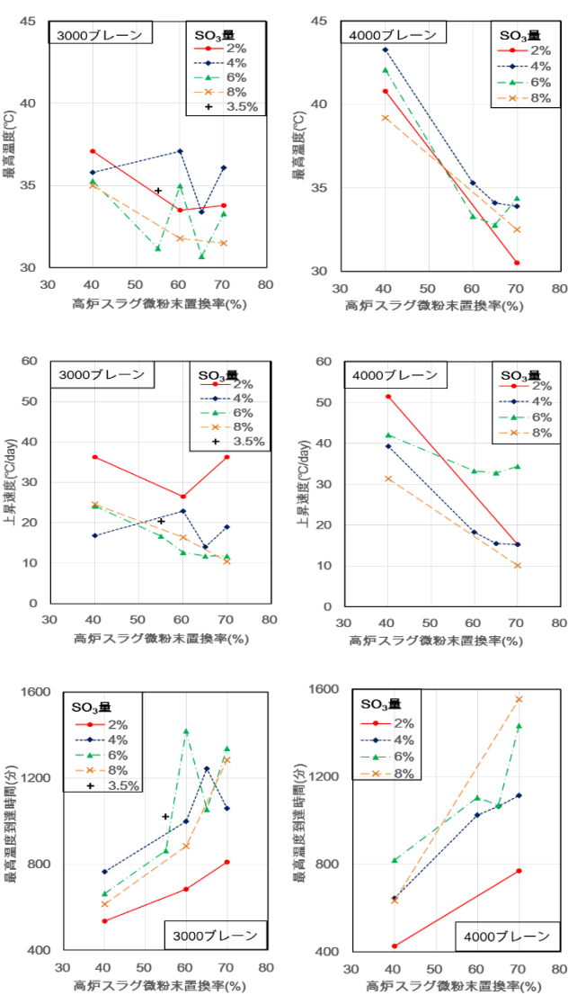
図-3 モルタル試験による発熱性状
