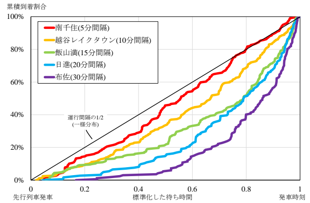
図-1 普通列車停車駅の累積到着割合
