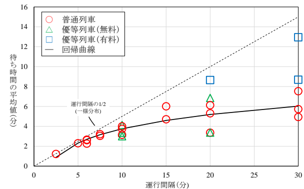
図-3 運行間隔と乗車待ち時間の平均値との関係
