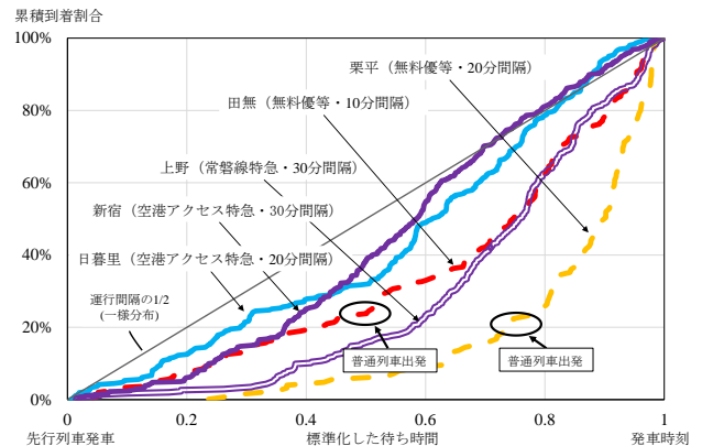
図-2 優等列車停車駅の累積到着割合
