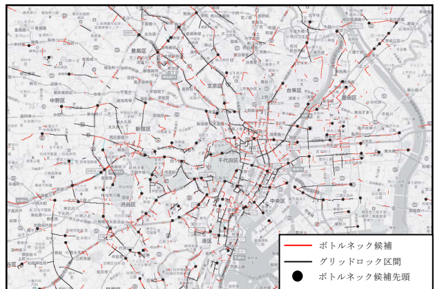
図-3 ボトルネックの抽出結果
